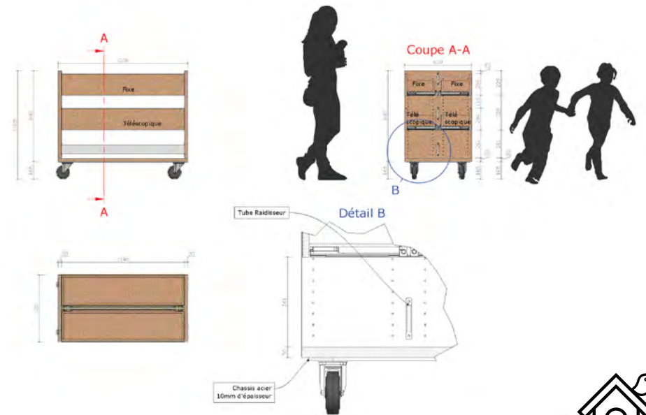
Dessin d'exécution
